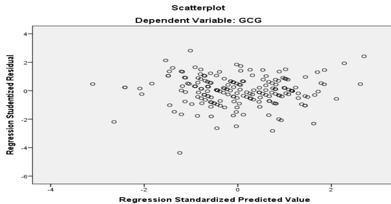
Gambar 1 Uji Heteroskedastisitas
